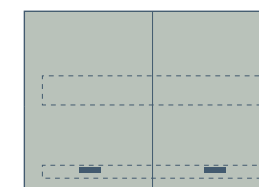
PENSILE SCOLAPIATTI 2 ANTE U 06 15 cm 90x37x60 H
