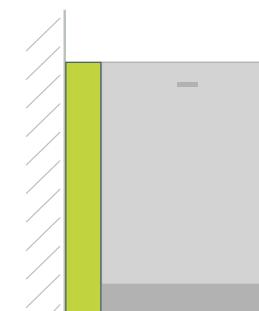
FASCIA TAMPONAMENTO Da utilizzare con basi inizio o fine composizione addossate al muro. U 06 FAB cm 5/10x1,8x87 H
