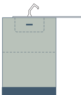
BASE PER LAVELLO 1 ANTA U 06 27 cm 60x58x87 H
