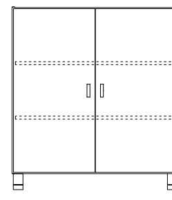
M 18 19 2 ANTE cm 104x41x114 H
