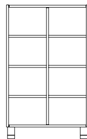
M 18 145 8 VANI A GIORNO cm 70x41x114 H
