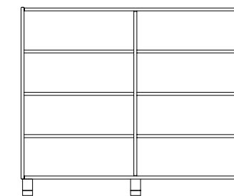
M 18 162 8 VANI A GIORNO cm 138x41x114 H
